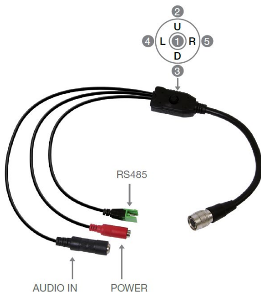
CV503、CV506、CV344、CV346 用 I/O ケーブル(同梱)
